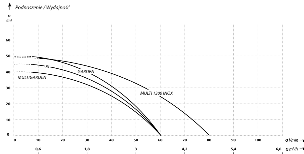
POMPA GARDEN Z OSPRZĘTEM HYDROFOROWYM
