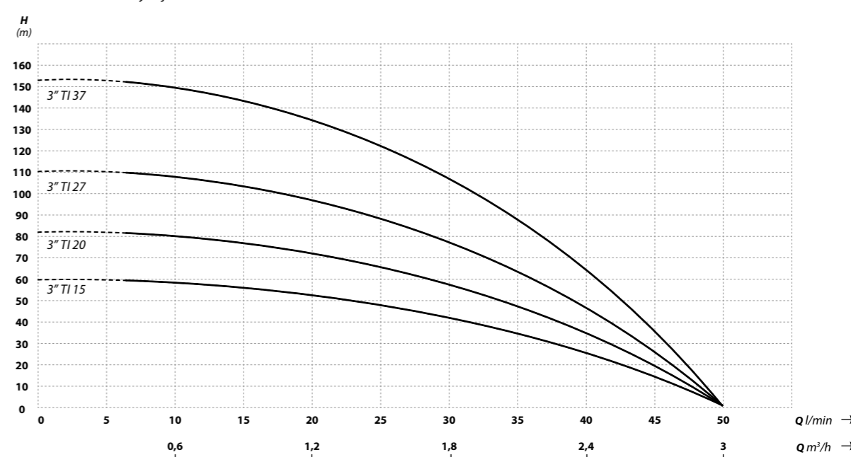
↑ Podnoszenie / Wydajność
