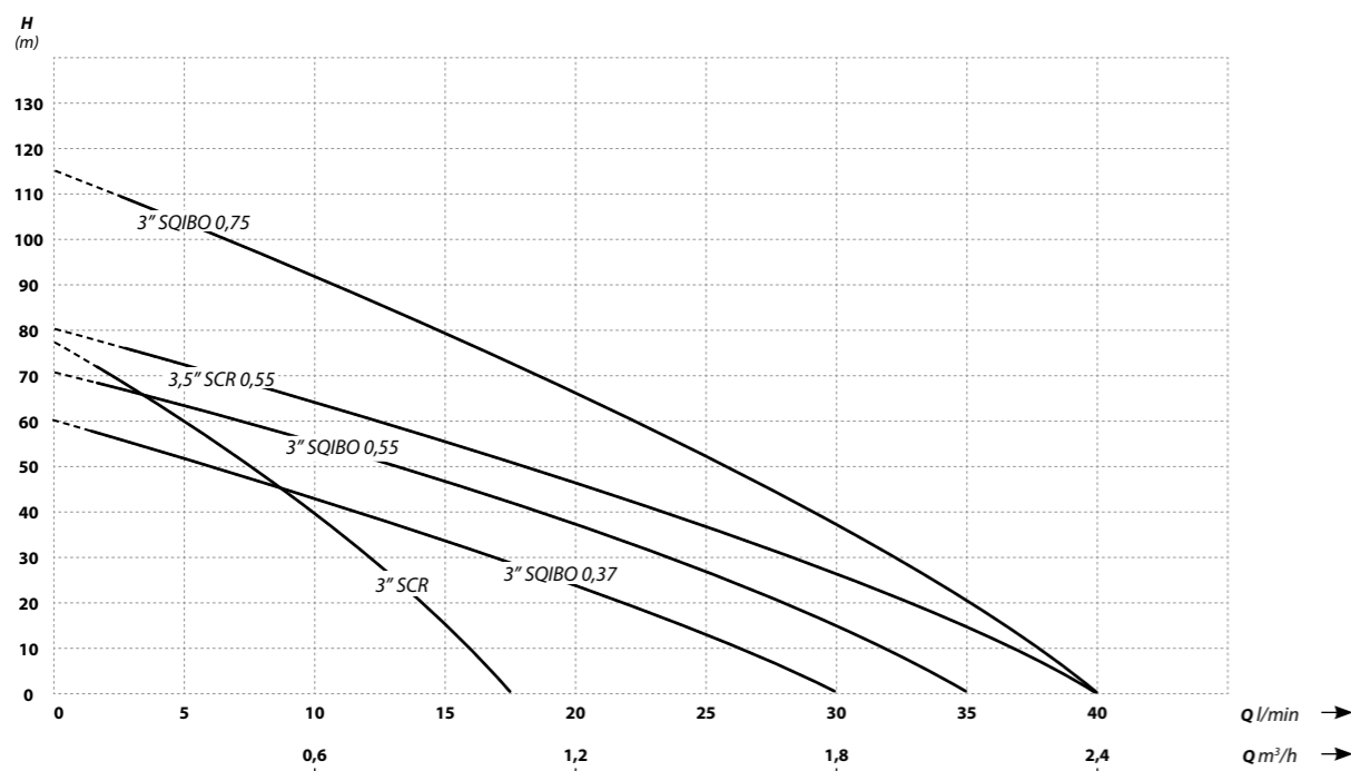
↑ Podnoszenie / Wydajność
