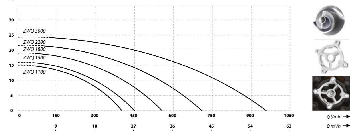
↑ Podnoszenie / Wydajność H (m)
