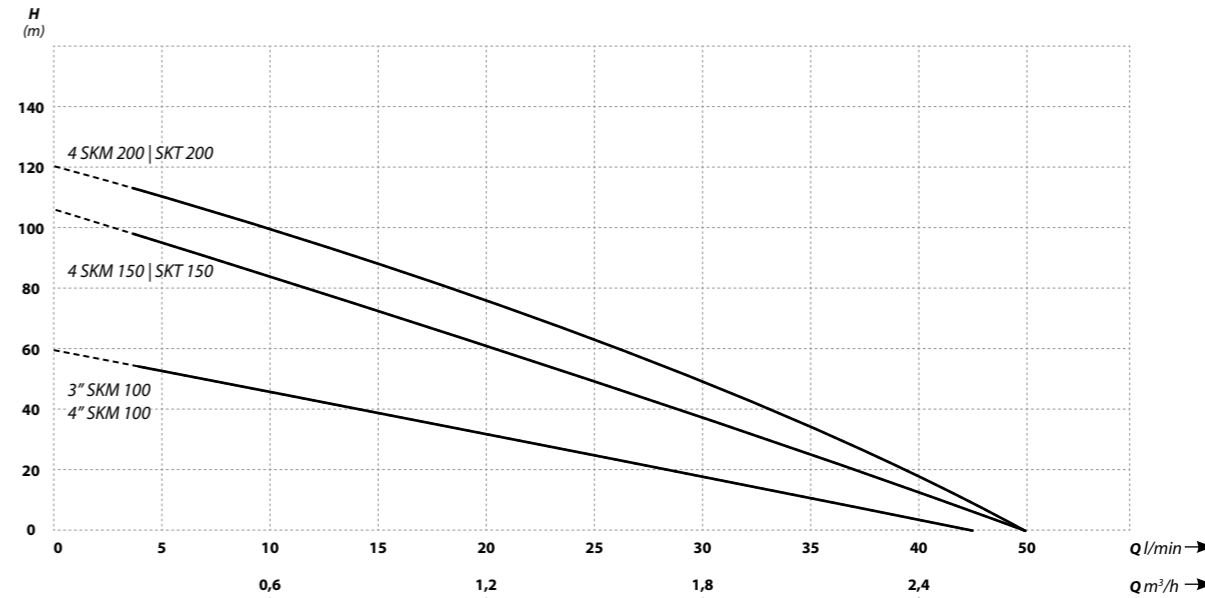
↑ Podnoszenie / Wydajność
