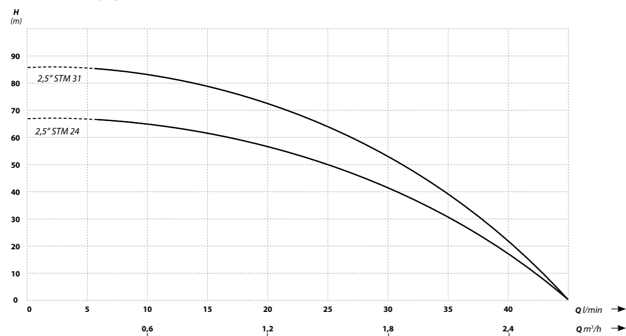
↑ Podnoszenie / Wydajność
