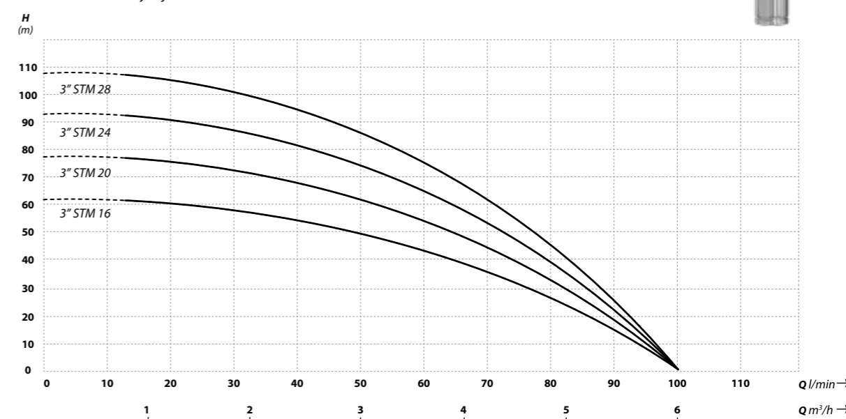
↑ Podnoszenie / Wydajność
