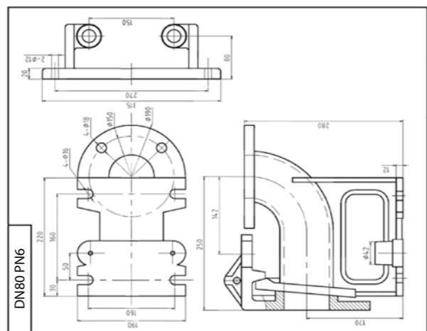
Stopa sprzęgająca
