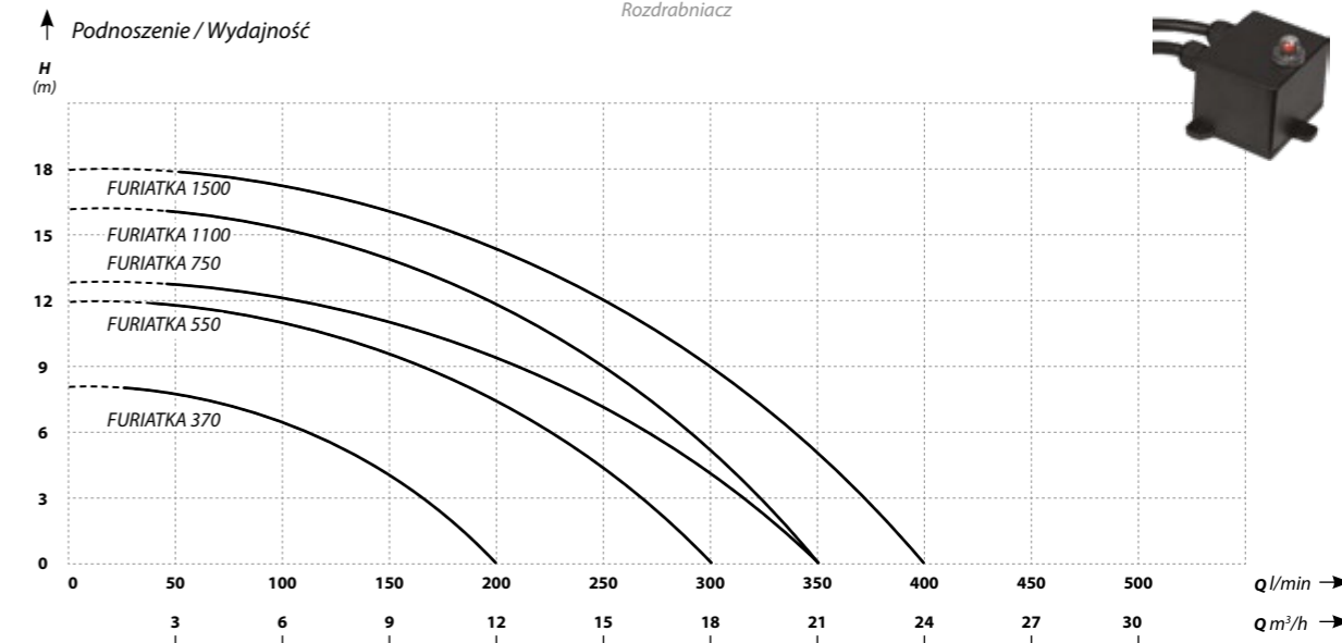
Rozdrabniacz
