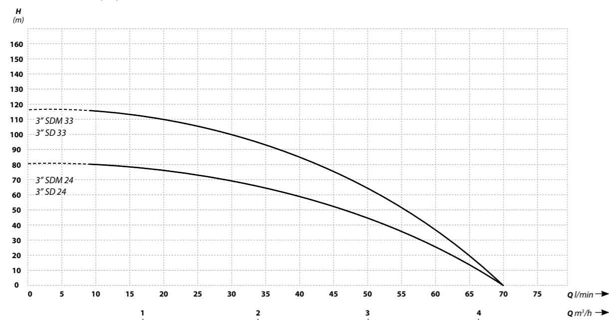
↑ Podnoszenie / Wydajność
