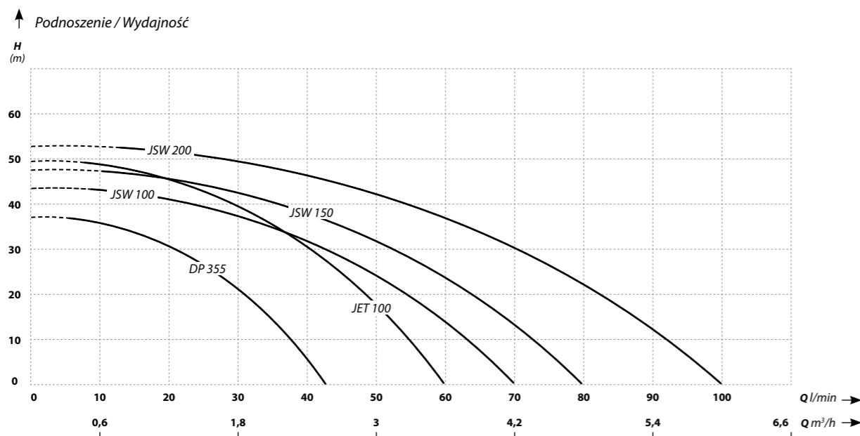
POMPA DP 355 Z OSPRZĘTEM HYDROFOROWYM
